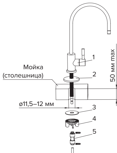
Рис. 4. Схема установки крана для чистой воды
