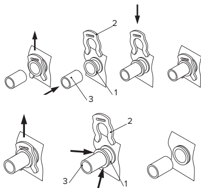
Рис. 3. Схема установки узла подключения
