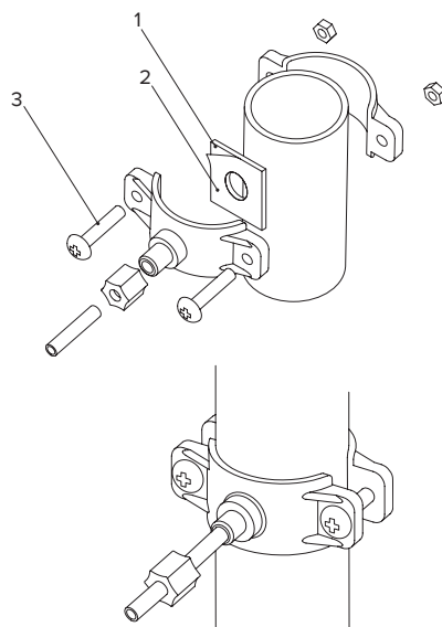
Рис. 5. Установка дренажного хомута
