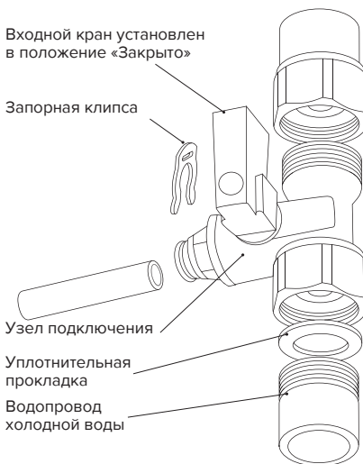
Рис. 3. Схема установки узла подключения
